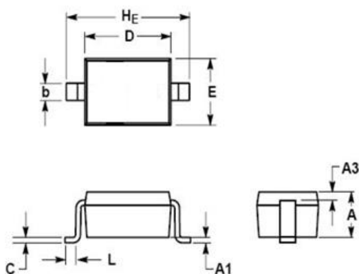
SOD323
