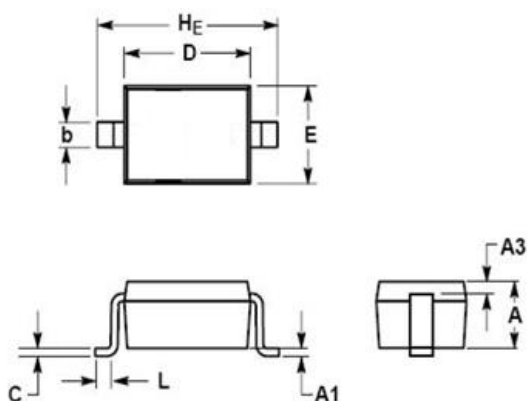
SOD323
